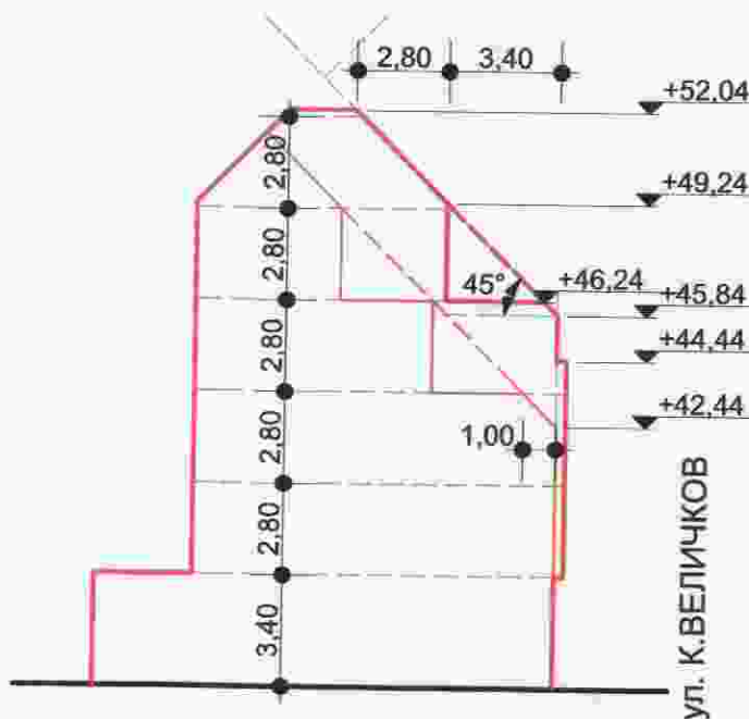
РАЗРЕЗ 1-1
